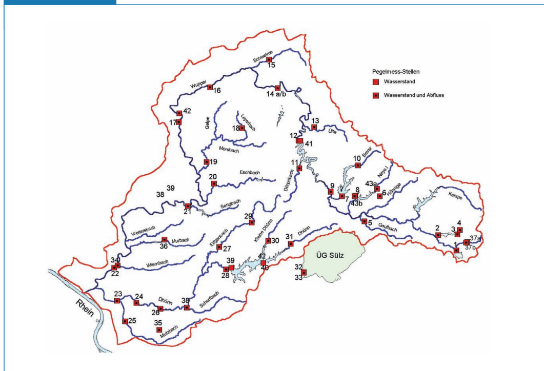
▶ Abb. 3.1.1.4-1 Übersicht über die Lage der Pegel im Einzugsgebiet der Wupper
