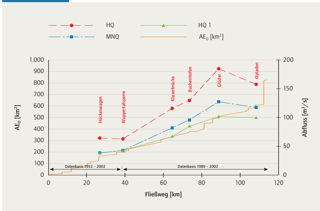
▶ Abb. 3.1.6-2 Hydrologischer Längsschnitt der Wupper für MHQ, HQ und HQ1
