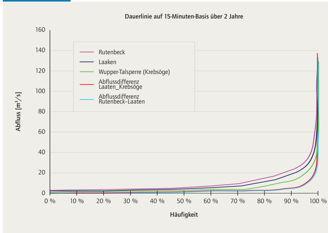
▶ Abb. 4.1.2.1-5 Normierte Dauerlinien Pegel Krebsöge und Zwischengebiete
