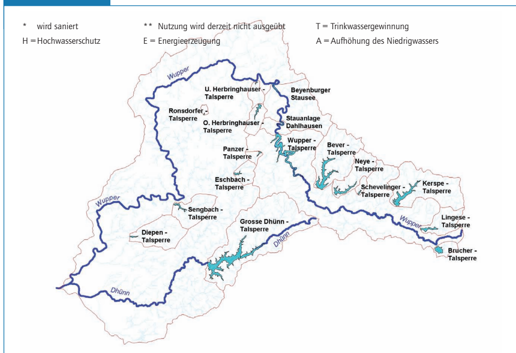
► Abb. 3.1.6-1 Talsperren mit Einzugsgebieten im Wuppereinzugsgebiet
