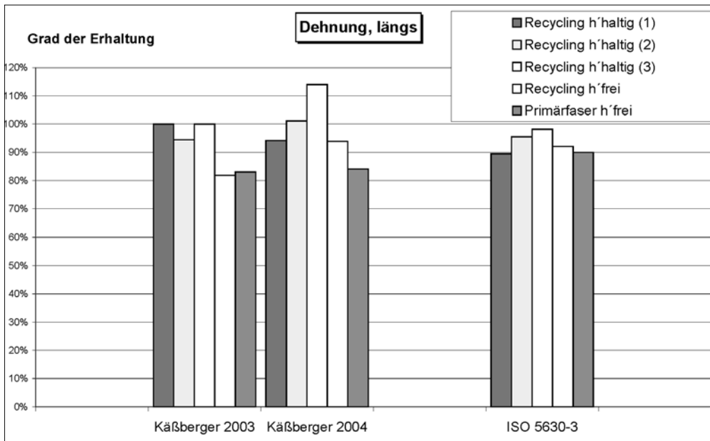
Bild 2: Dehnung längs
