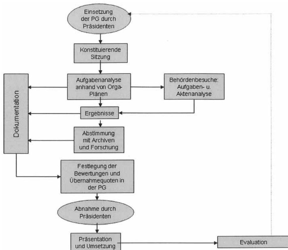
Abbildung 3: Ablaufdiagramm Archivierungsmodell
