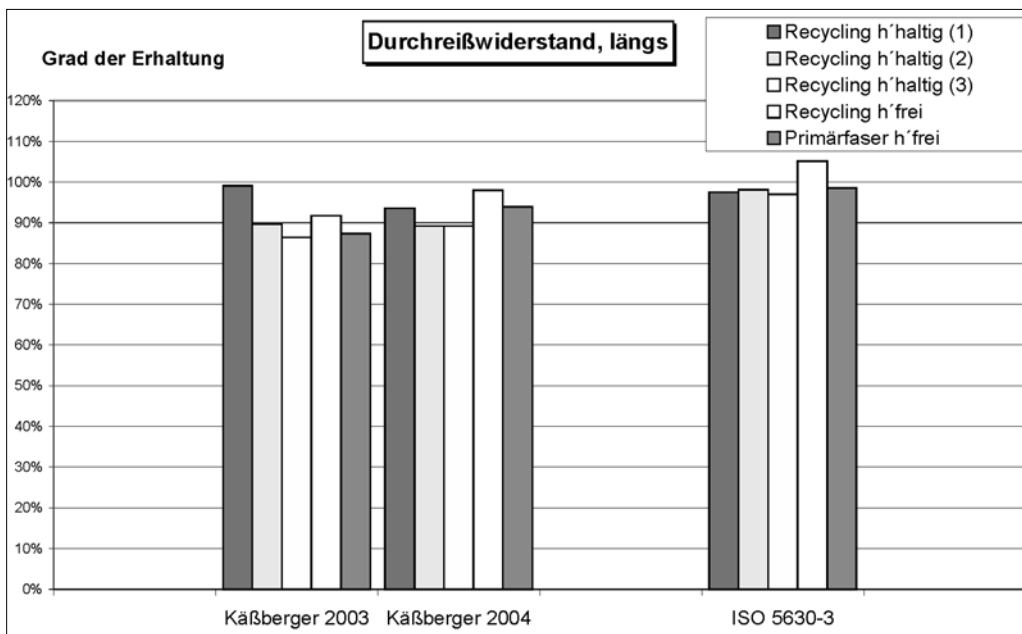
Bild 3: Durchreißwiderstand längs
