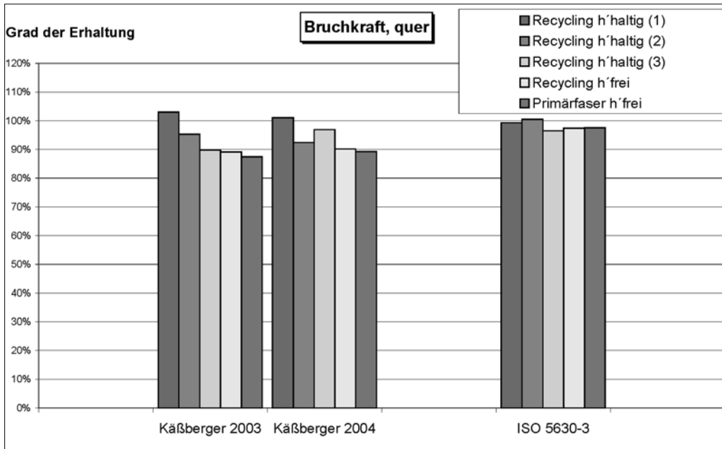
Bild 1: Bruchkraft quer
