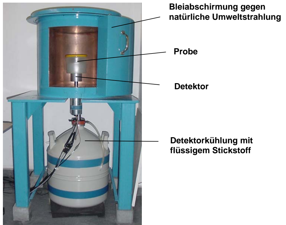
Abb. 2.4: Messplatz für Gammaspektrometrie
