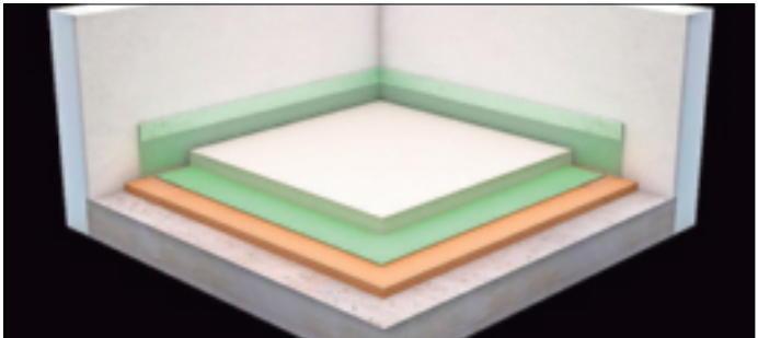
Fachgerechter Bodenaufbau für wirksamen Trittschallschutz. Foto: djd/ VDPM
