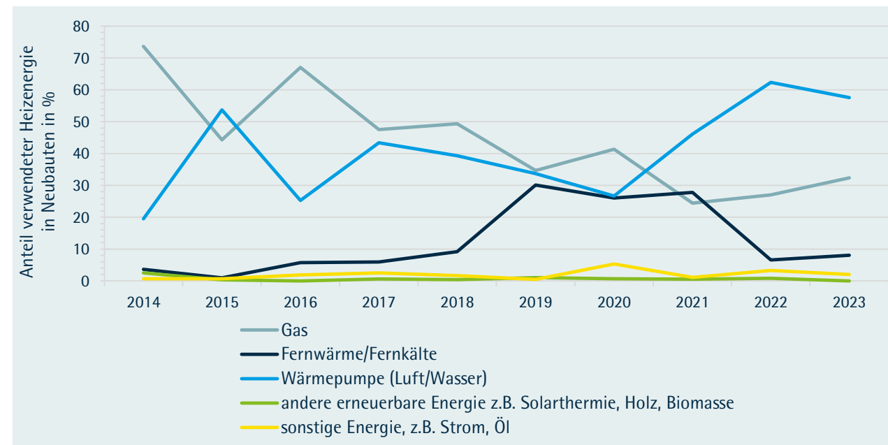
Abbildung 27: Entwicklung Anteil primärer Heizenergie im Neubau von Wohngebäuden und sonstigen Gebäuden in Prozent
