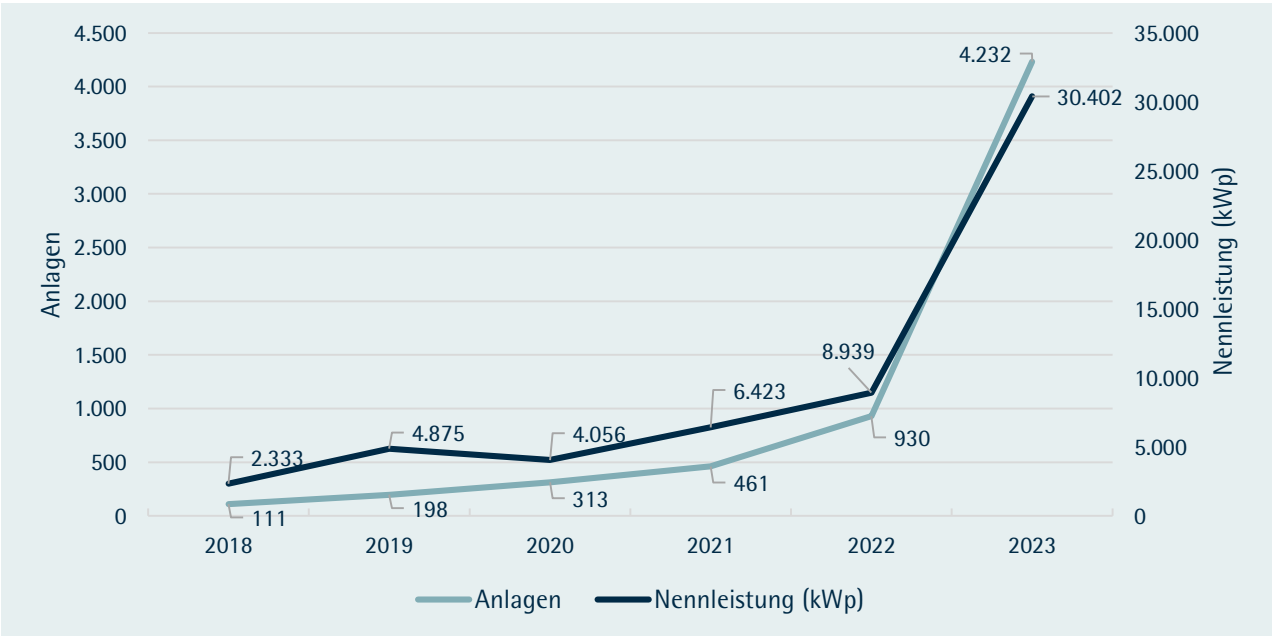
Abbildung 69: Entwicklung der installierten Photovoltaikanlagen in Essen
