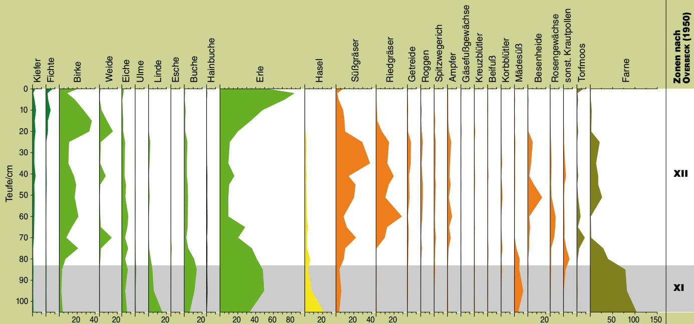
Abb. 6: Pollendiagramm der Bohrung Krähenfuhl
