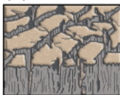
Prismengefüge
