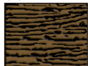
Plattengefüge
