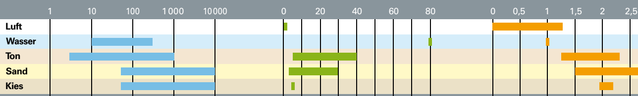
Geoelektrik – elektrischer Widerstand [ \Omega\text{m} ]
