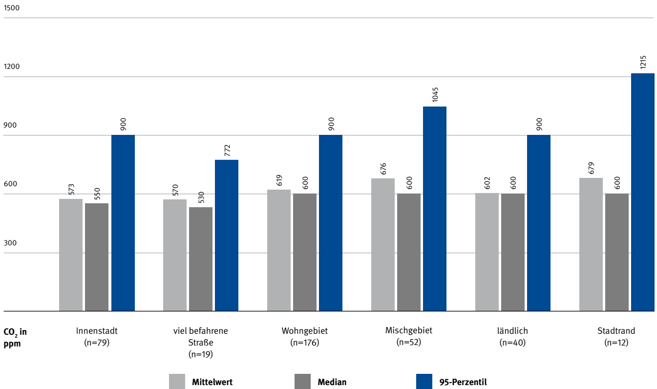
Abb. 24: Grundbelastung von CO 2 vor Unterrichtsbeginn in Abhängigkeit von der Lage der Schule
