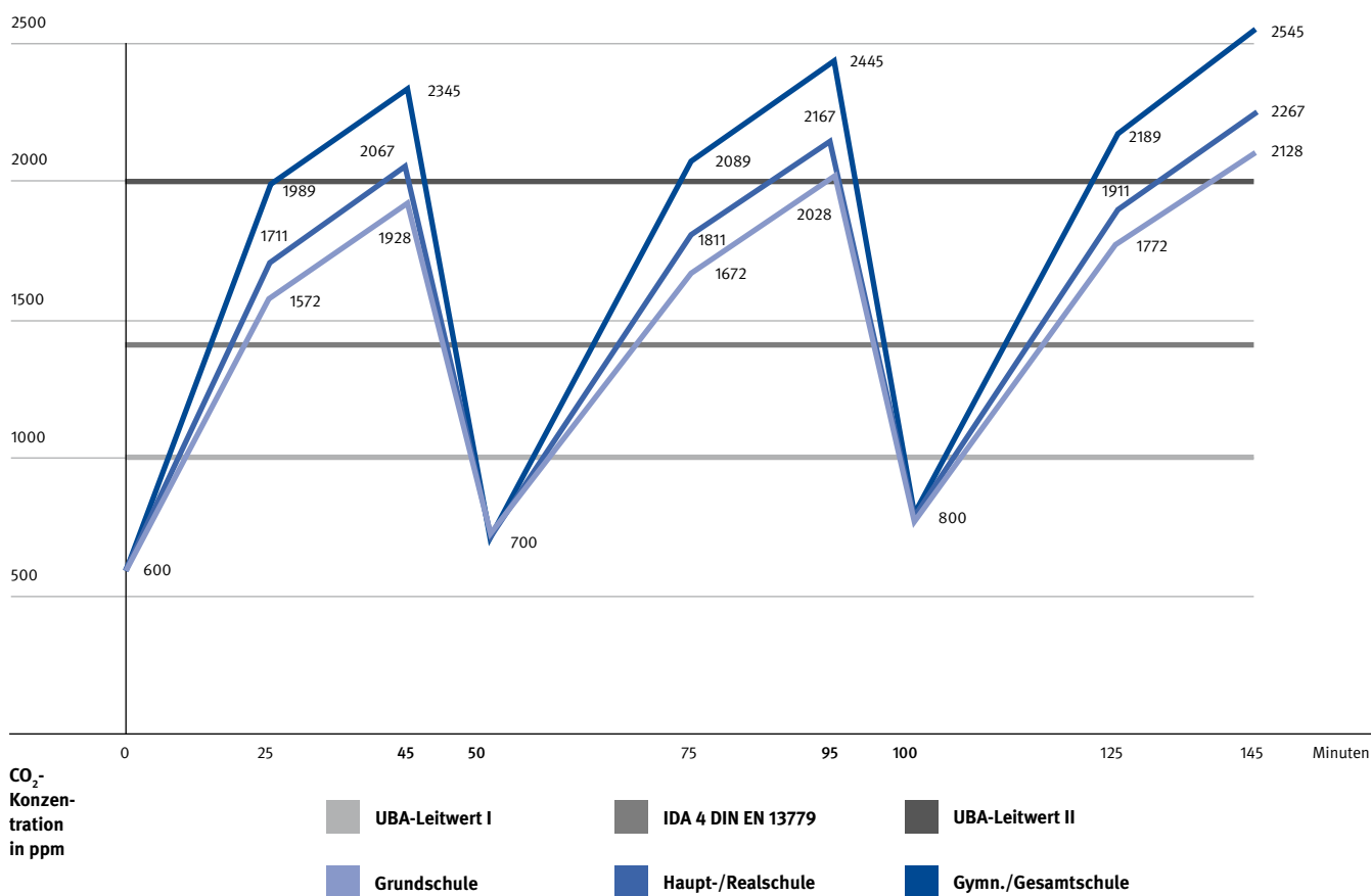
Abb. 43: Modellhafte Darstellung von CO 2 -Konzentrationen im Unterricht verschiedener Schulformen in Anlehnung an die ermittelten 95-Perzentilwerte für die CO 2 -Anstiege pro Raumnutzer und Kipplüftungsintervention im Winterszenario nach 25 Minuten Unterrichtszeit bei einer Raumnutzerzahl von 25
